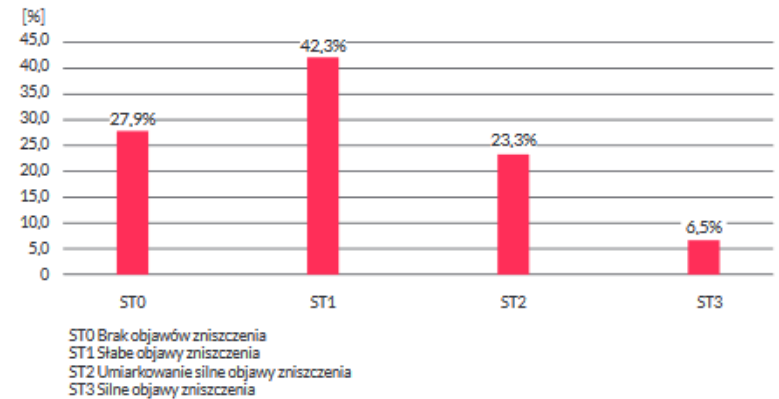
STAN TECHNICZNY PRZEBADANYCH OBIEKTÓW
